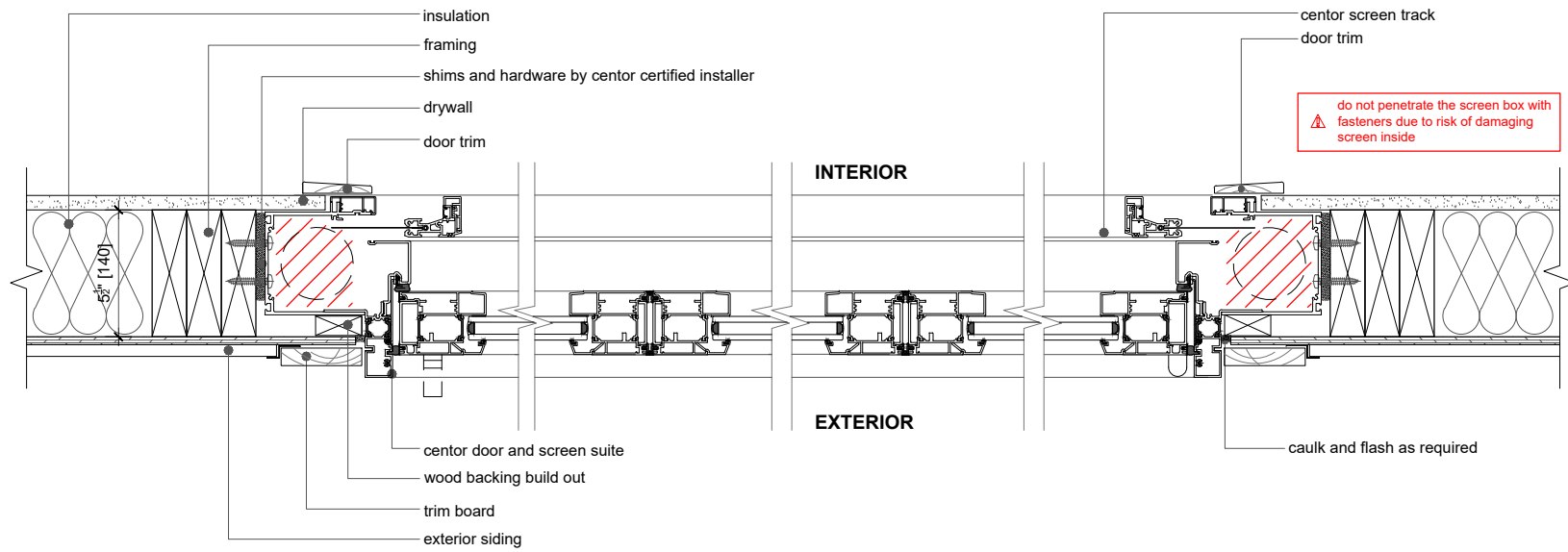
1 jamb detail plan
